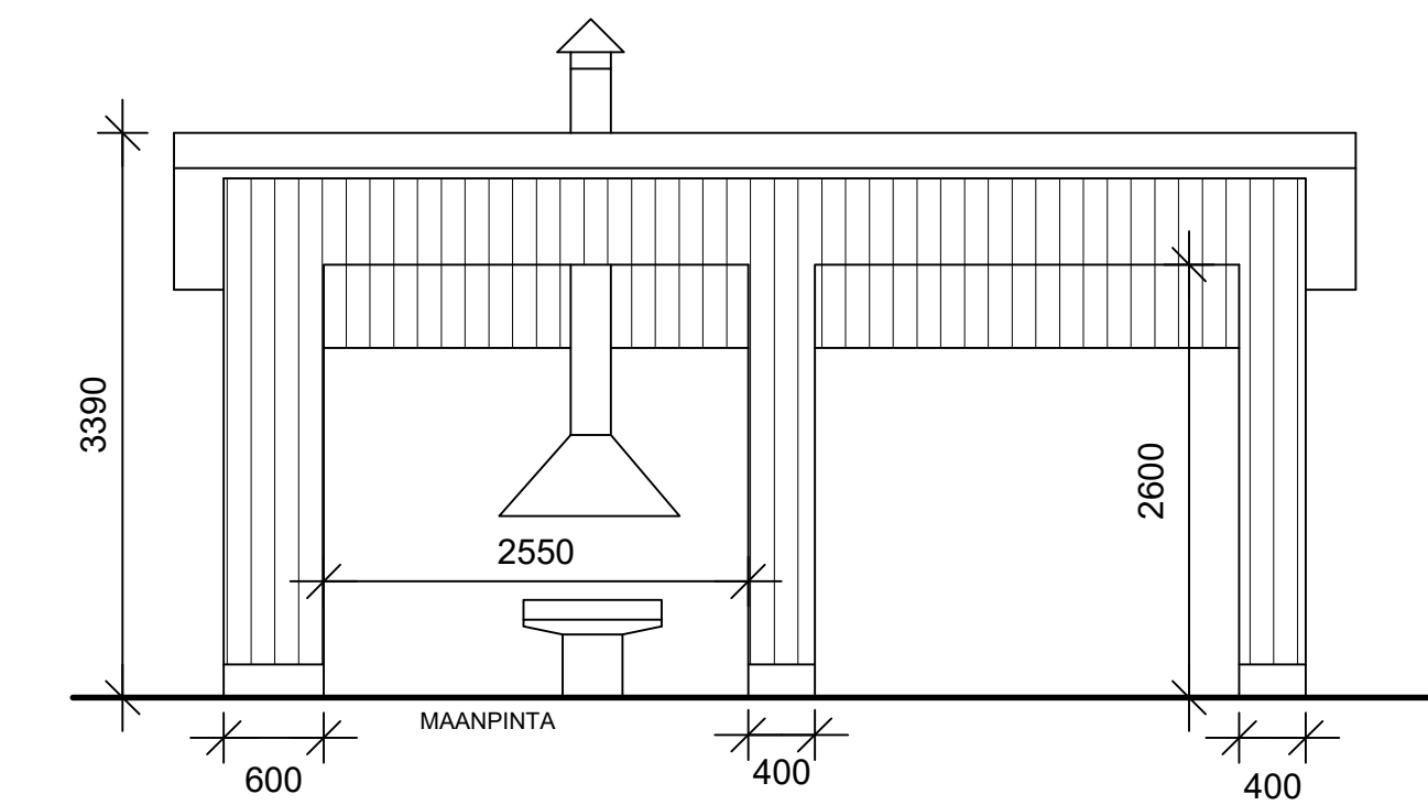
Julkisivu länteen
