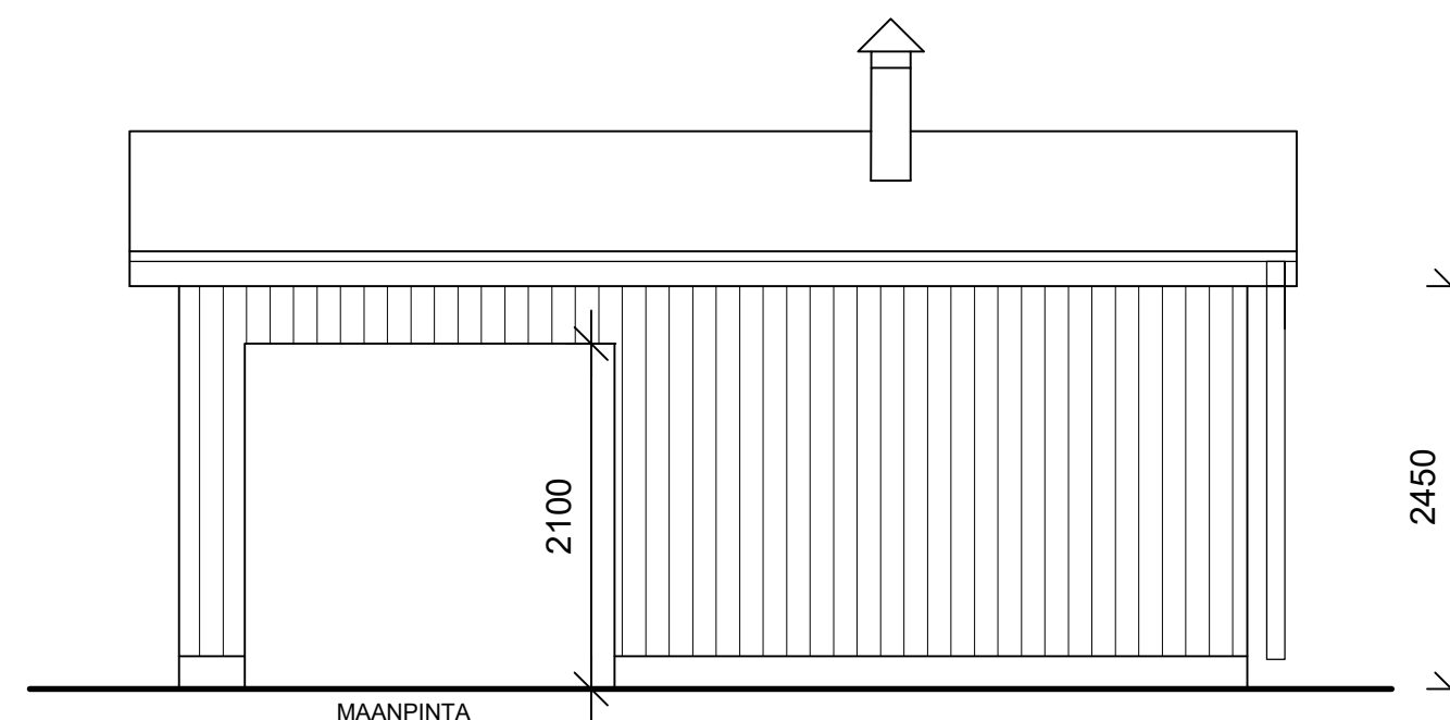
Julkisivu itään
