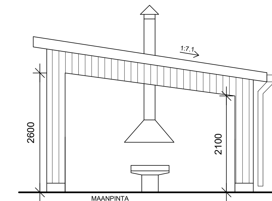
Julkisivu etelään
